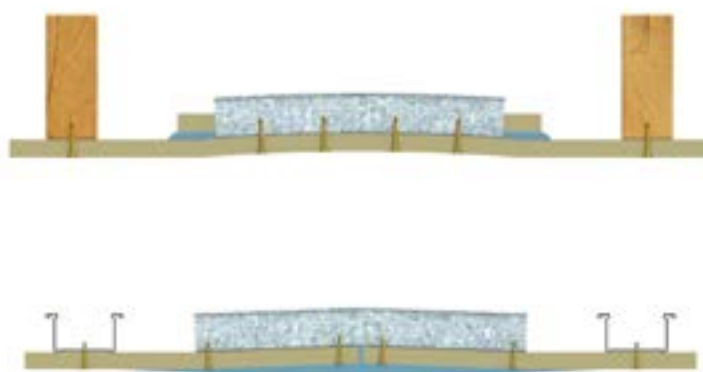
■ STITCHING BATTENS
